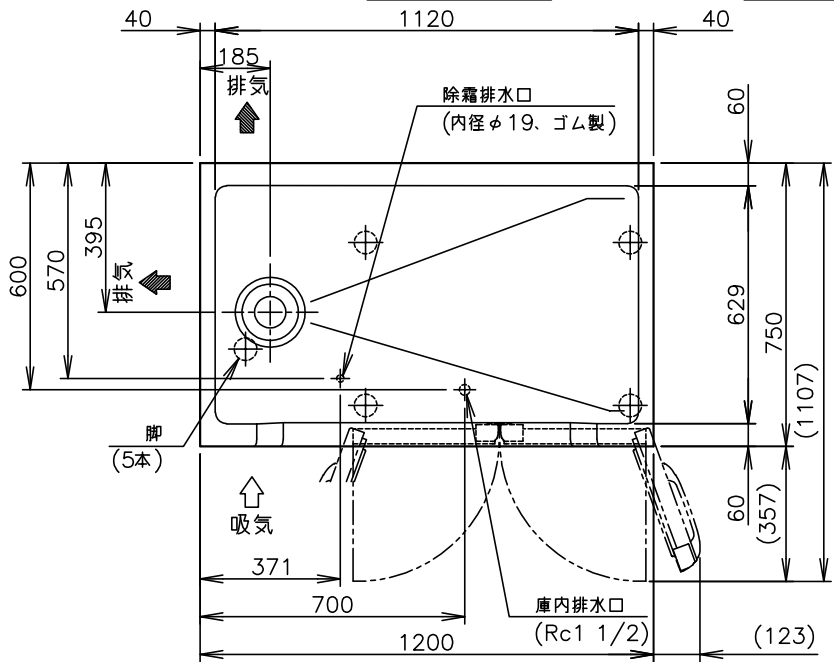
A矢視図(1/10)
