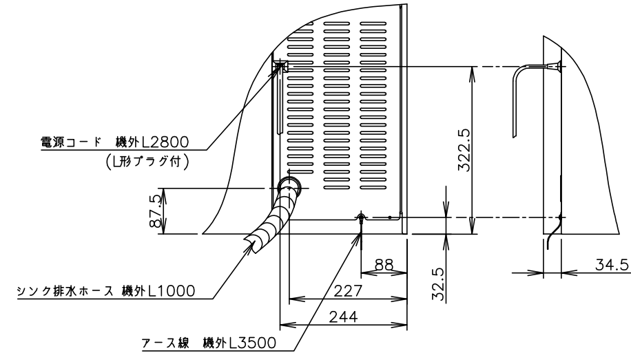
A矢視図(1/10)
