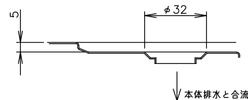
K-K断面(5/1)
