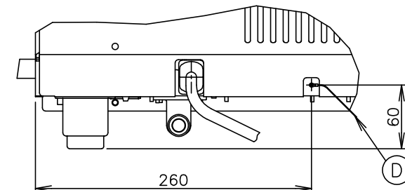
背面図(2/1)
