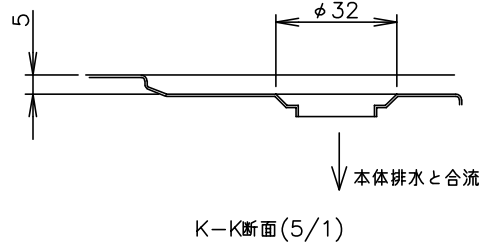
K-K断面(5/1)
