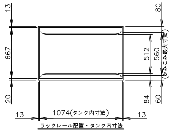
ガスプースター組込み図
