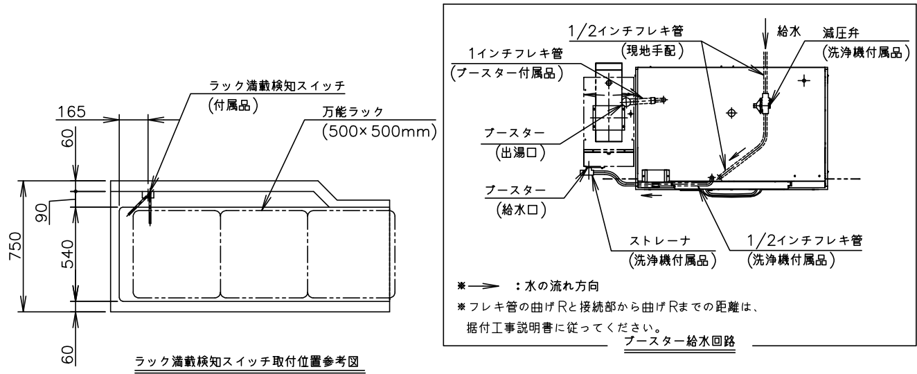
ラック満載検知スイッチ取付位置参考図
