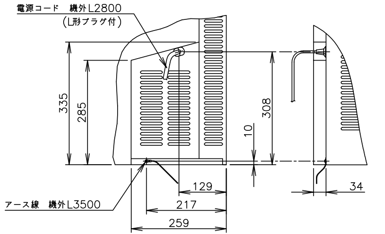
A矢视图 (1/10)
