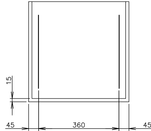
ラックレイアウト図
